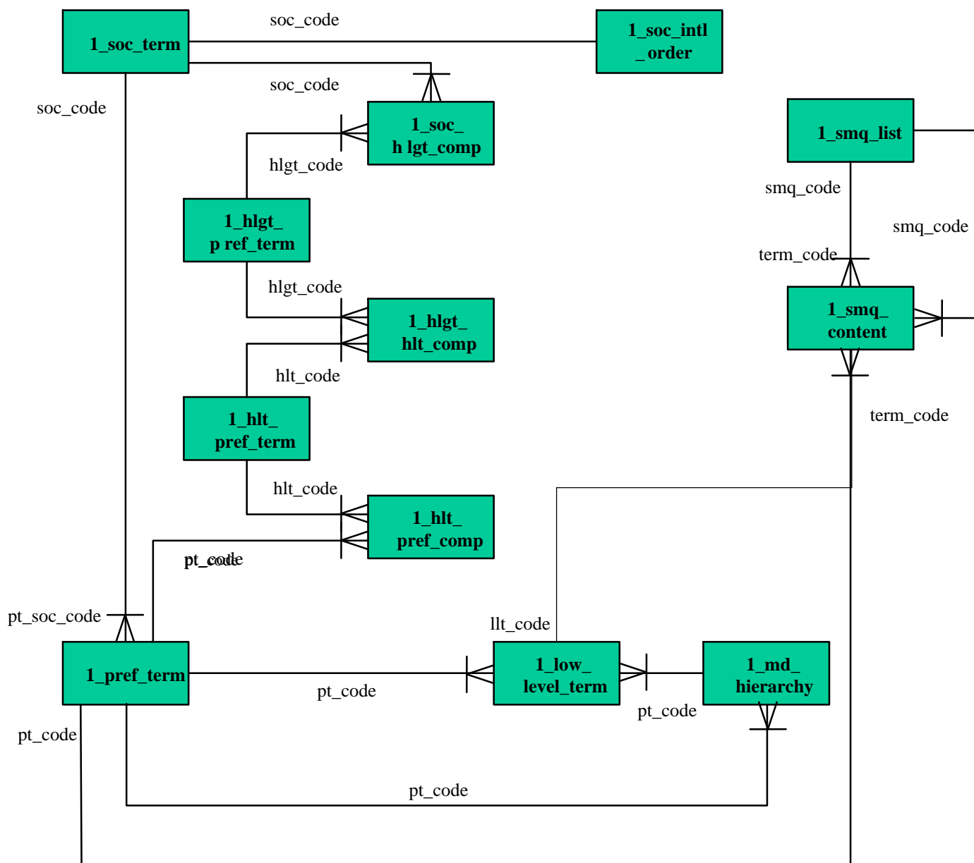
Рисунок 6-1. Модель данных MedDRA
