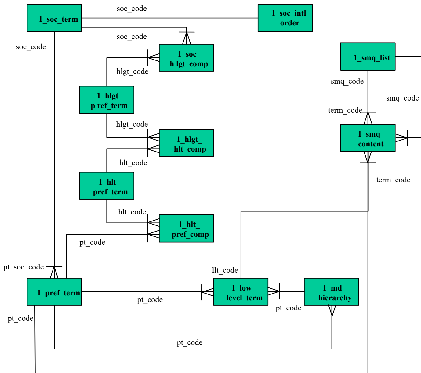
6-1. ábra. MedDRA adatmodell
